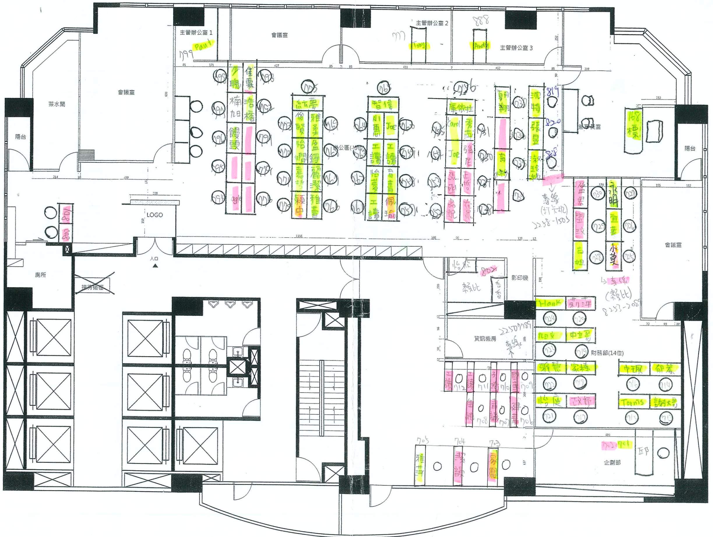
學習王辦公室 隔間尺寸圖 S:1/100 cm date:2020.10.10
